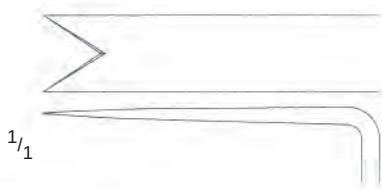
21-1397-45 22 cm/8 3 / 4 " Spina nasalis-Haken Nasal Spine Retractor Separador para spina nasalis Ecarteur pour spina nasalis 45 x 10 mm
